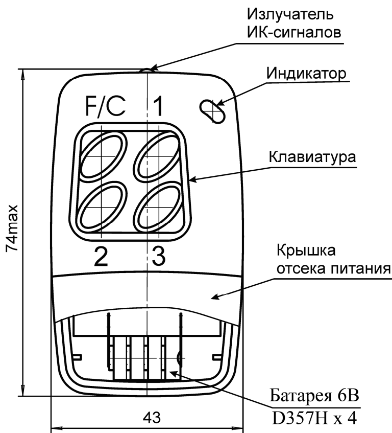
Рис. 1 Внешний вид пульта и габаритные размеры.
